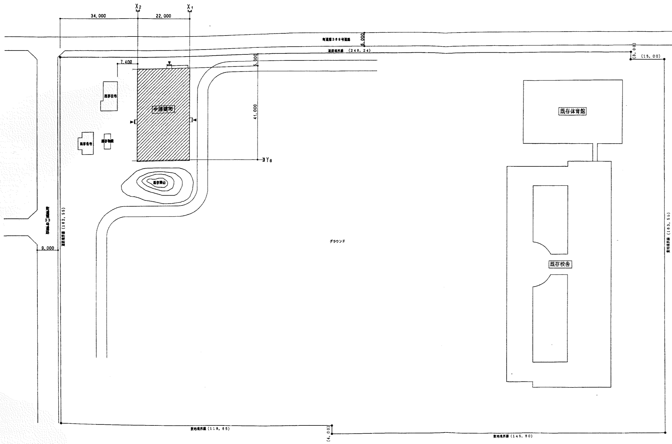
配置図 1:500
