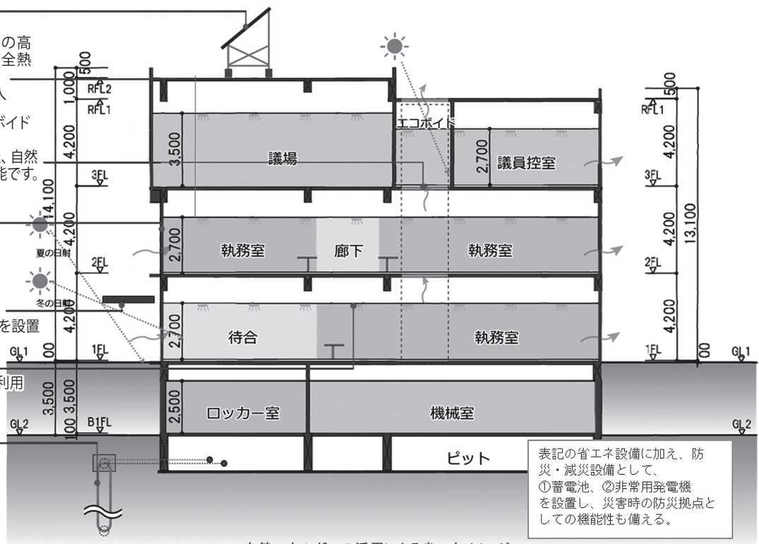
自然エネルギーの活用による省エネイメージ
